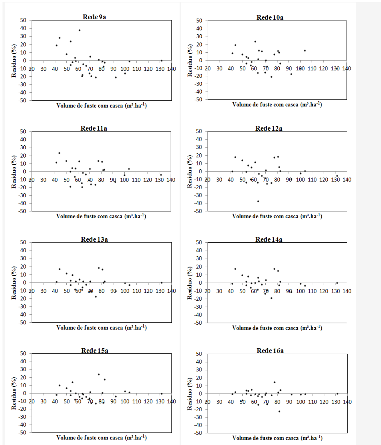
Figura 2.5 – Distribuição dos resíduos percentuais das redes neurais artificiais ajustadas para estimar os volumes de fuste com casca, em \text{m}^3.\text{ha}^{-1} , para um hectare de amostragem em um remanescente de Floresta Estacional Semidecidual em Curvelo, MG.
