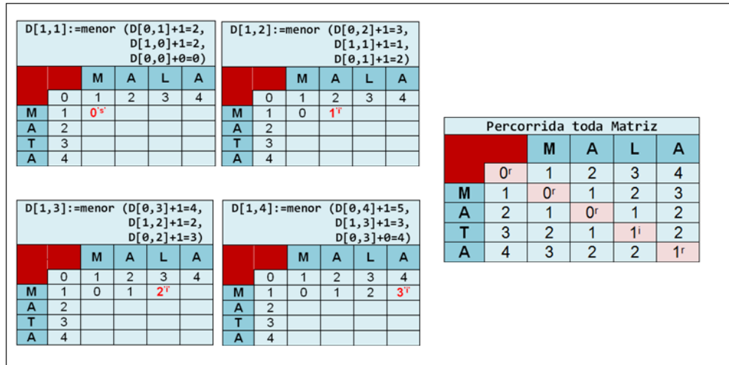
Figura 3 - Algoritmo Levenshtein
